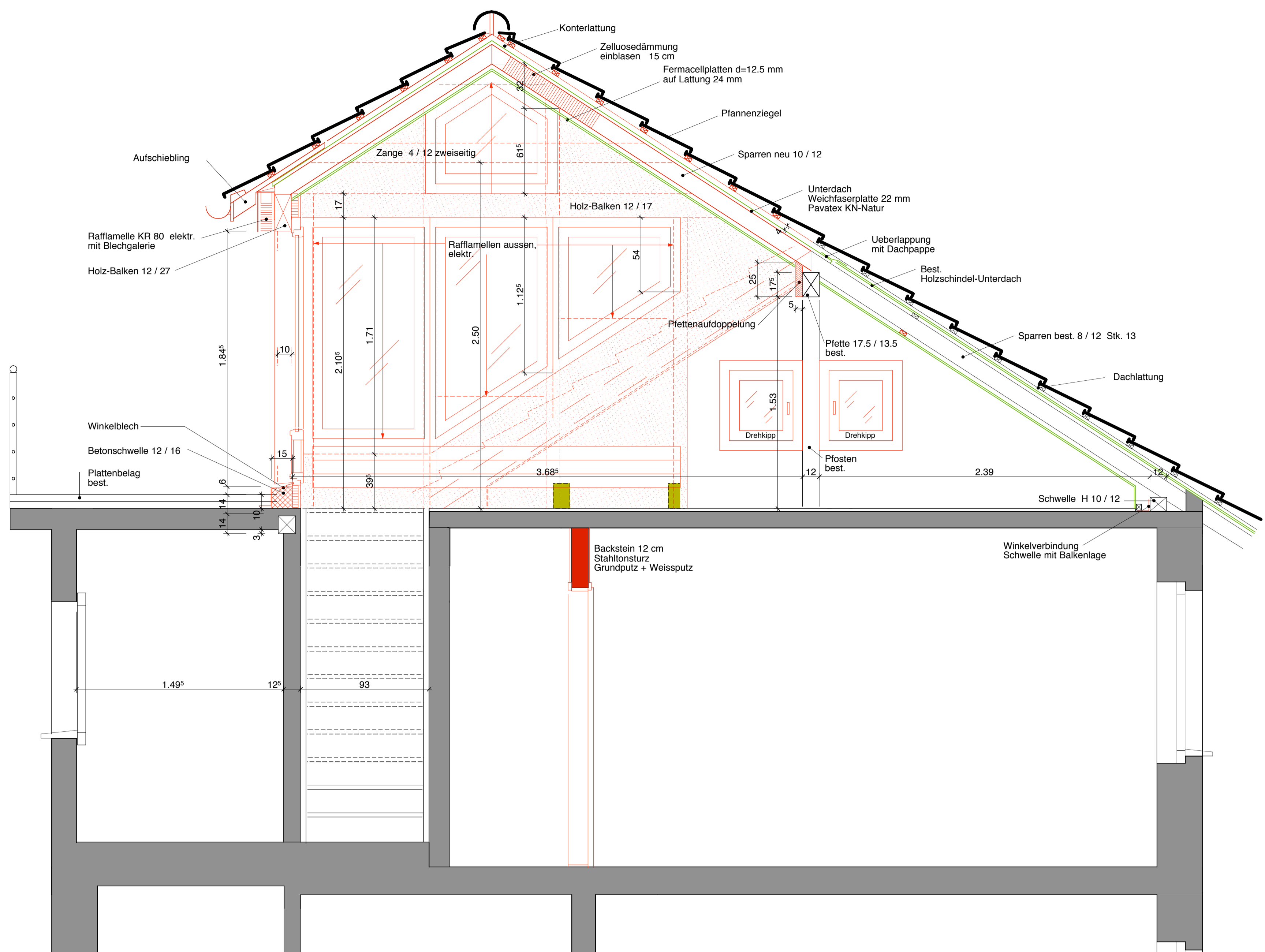
Schnitt A --- A
