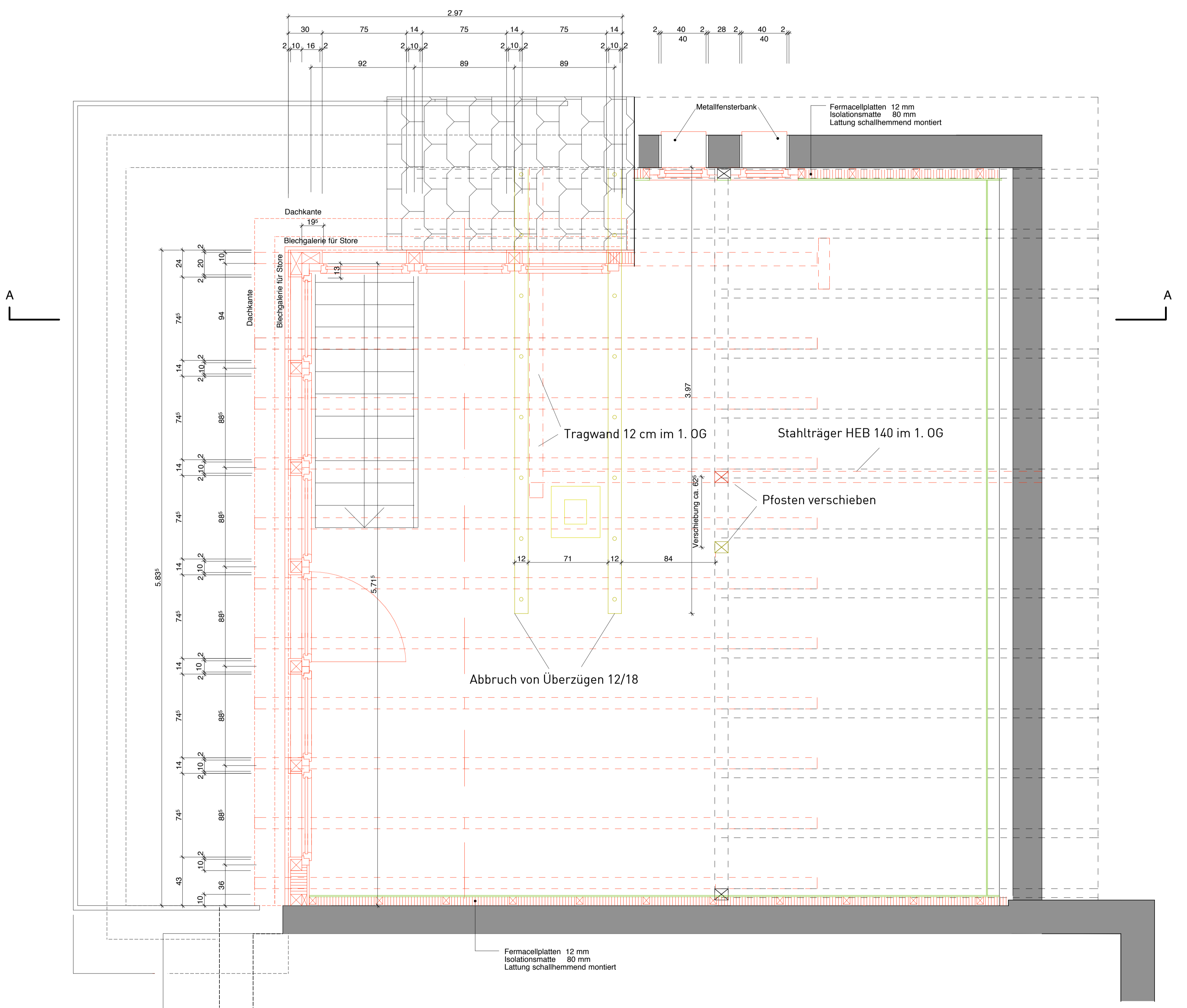
Grundriss Dachgeschoss
